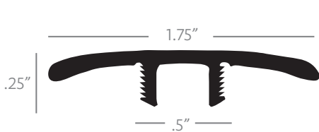
T-MOLD
