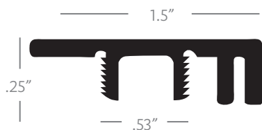
END CAP
